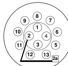
Podłączenie przewodów w gnieździe 13-biegunowym
