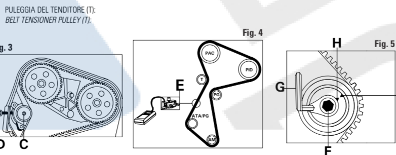
FIGURA 3 Allentare il bullone di bloccaggio C e inserire l'apposito attrezzo di tensionamento D, avvitandolo fino alla corretta tensione; serrare quindi il bullone di bloccaggio C. FIGURA 4 Inserire l'apposito attrezzo di misura del tensionamento E, nel punto indicato, ed agire sul tendicinghia fino ad un valore compreso tra 42.3 e 51.7 unità SEEM (per modello Renault Kangoo); 37 unità SEEM (per modello Renault Espace); 61 ± 5 Hz (per modello Volvo S40). FIGURA 5 Allentare il bullone di bloccaggio F e ruotare in senso antiorario il tendicinghia utilizzando la chiave esagonale G, fino ad allineare le tacche di fase H ed I; serrare, quindi, il bullone di bloccaggio F.
