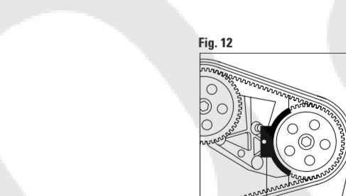
FIGURA 11 Controllare il corretto allineamento delle tacche di fase Q. FIGURA 12 Inserire l'apposito attrezzo di bloccaggio della puleggia della pompa di iniezione R.
