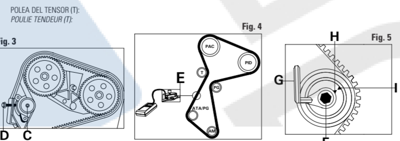
FIGURA 3 Aflojar el tornillo de fijación C. Insertar la herramienta específica D para tensado de correa, atomillándola hasta obtener la tensión correcta. Por último, apretar el tornillo de fijación C. FIGURA 4 Insertar la herramienta apropiada para medición de la tensión E en el punto indicado, y actuar sobre el tensor de la correa hasta conseguir un valor de tensión comprendido entre 42.3 y 51.7 unidades SEEM (Para modelos Renault Kangoo), 37 unidades SEEM (Para modelo Renault Espace), y de 61 ± 5 Hz (Para modelos Volvo S40). FIGURA 5 Aflojar el tornillo de fijación F. Girar el tensor de correa sobre el excéntrico de regulación G en sentido contrario a las agujas del reloj utilizando para ello la llave hexagonal G hasta alinear las muescas de fase H y I. Por último, apretar el tornillo de fijación F.
