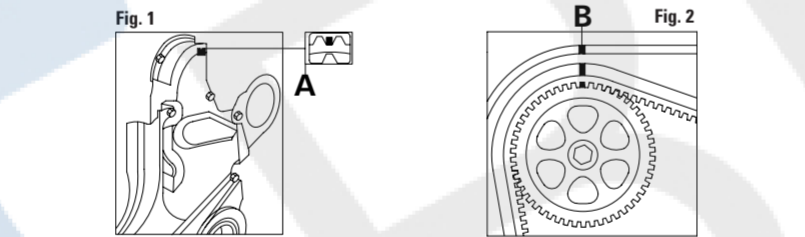
FIGURA 1 Verificar que la marca de puesta a tiempo este en línea con la marca del cárter de la distribución A. FIGURA 2 Verificar la correcta alineación de las marcas de puesta en fase B.
