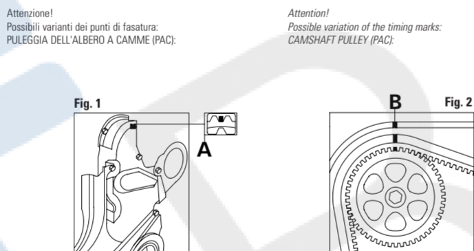
FIGURA 1 Controllare il corretto allineamento della tacca di fasatura, verificando che risulti allineata al carter distribuzione A. FIGURA 2 Controllare il corretto allineamento delle tacche di fase B.
