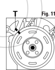
FIGURA 11 Controllare il corretto allineamento delle tacche di fase T.
