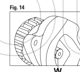
FIGURA 14 Allentare il bullone di bloccaggio W posto sul retro del tendicinghia del contralbero.
