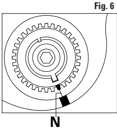
FIGURA 6 Verificar la correcta alineación de las marcas de fase N.
