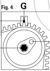
FIGURA 4 Aflojar el tornillo de fijación D. Girar el tensor de la correa sobre el excéntrico de regulación E, en sentido de las agujas del reloj hasta lograr que el indicador F quede alineado con la muesca de fase G. Por último, apretar el tornillo de fijación D.
