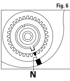
FIGURA 6 Verificar la correcta alineación de las marcas de fase N.
