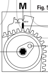
FIGURA 4 Aflojar el tornillo de fijación D. Girar el tensor de la correa sobre el excéntrico de regulación E, en sentido de las agujas del reloj hasta lograr que el indicador F quede alineado con la muesca de fase G. Por último, apretar el tornillo de fijación D. FIGURA 5 Aflojar el tornillo de fijación I. Girar el tensor de la correa sobre el excéntrico de regulación H en sentido de las agujas del reloj. Luego, alinear el indicador L con la muesca de fase M. Por último apretar el tornillo de fijación I.
