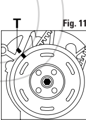
FIGURA 11 Controllare il corretto allineamento delle tacche di fase T. FIGURA 12 Controllare il corretto allineamento delle tacche di fase U. FIGURA 13 Controllare il corretto allineamento delle tacche di fase V.
