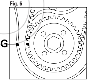
FIGURA 6. Controllare il corretto allineamento delle tacche di fase G. FIGURA 7. Inserire l'apposito attrezzo di bloccaggio del volante H.
