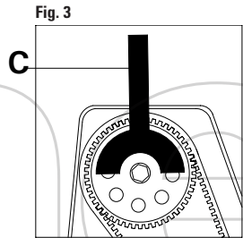
FIGURA 1. Inserire l'apposito attrezzo di comparazione A, sul cilindro N° 1. FIGURA 2. Controllare il corretto allineamento delle tacche di fase B. FIGURA 3. Inserire l'apposito attrezzo C, per mantenere l'ingranaggio in tensione. FIGURA 4. Inserire l'apposito attrezzo di bloccaggio dell'albero a camme D.
