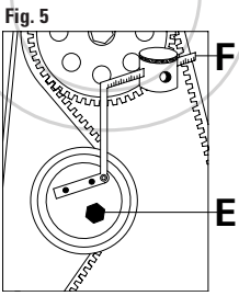
FIGURA 5. Aflojar el tornillo de fijación E, e insertar la herramienta especial de tensado de correa con su relativo peso (65mm o 70mm). Verificar que el brazo de la herramienta se mantenga en posición horizontal. Por último, apretar el tornillo de fijación E.
