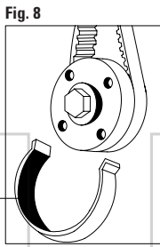
FIGURA 6 Inserire l'apposito attrezzo di bloccaggio del volano P. FIGURA 7 Controllare il corretto allineamento della tacca di fase Q. FIGURA 8 Inserire l'apposito attrezzo di bloccaggio della cinghia di distribuzione R.
