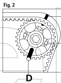
FIGURA 1 Inserire l'apposito attrezzo di bloccaggio dell'albero a camme A. Allineare i punti di fase B: i bulloni C non devono trovarsi all'estremità delle scanalature. FIGURA 2 Inserire l'apposito attrezzo di bloccaggio dell'albero a camme D. Allineare i punti di fase E. I bulloni F non devono trovarsi all'estremità delle scanalature.
