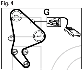
FIGURA 3 Allentare il bullone di bloccaggio E, ruotare il tendicinghia in senso antiorario tramite l'attrezzo di tensionamento F, fino alla corretta misura di tensione e serrare, quindi, il bullone di bloccaggio E. FIGURA 4 Inserire l'apposito attrezzo di misura del tensionamento, G, nel punto indicato, ed agire sul tendicinghia fino al valore di: 1° fase: 108 unità SEEM (per motori Peugeot / Fiat Ducato / Lancia) e 96-100 unità SEEM (per motori Citroen); 2° fase: 54 unità SEEM (per motori Peugeot / Fiat Ducato / Lancia) e 52-56 unità SEEM (per motori Citroen); 3° fase: 51-57 unità SEEM (per motori Citroen / Peugeot / Fiat Ducato / Lancia). Per motori Fiat e Lancia la tensione ha un valore compreso tra 48 e 55 unità SEEM.
