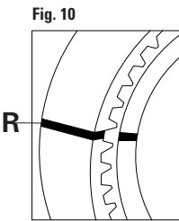
FIGURA 9 Inserire l'apposito attrezzo di bloccaggio della puleggia della pompa di iniezione Q. FIGURA 10 Controllare il corretto allineamento delle tacche di fase R. FIGURA 11 Inserire gli appositi attrezzi di bloccaggio della puleggia della pompa di iniezione S.
