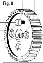
FIGURA. 9 Insertar la herramienta específica de inmovilización de la polea de bomba de inyección "O". FIGURA. 10 Verificar la correcta alineación de las marcas de puesta a punto "R". FIGURA. 11 Insertar las herramientas específicas para inmovilizar la polea de la bomba de inyección "S".
