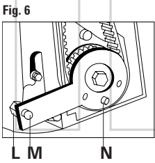
FIGURA. 6 Desmontar el tornillo de la bomba de aceite L, y en su lugar, instalar el prisionero de la herramienta de inmovilización M. Rotar el cigüeñal hasta alcanzar el PMS del cilindro N° 1 y verificar la correcta posición de la marca de la polea del cigüeñal N. FIGURA. 7 Insertar la herramienta especial de inmovilización del cigüeñal O. FIGURA. 8 Insertar la herramienta específica para inmovilizar el volante motor P.
