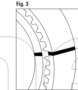
FIGURA. 1 Verificar la correcta alineación de las marcas de puesta en fase A. FIGURA. 2 Verificar la correcta alineación de las marcas de fase; 7 dientes de adelanto con respecto a la marca de fase ubicada sobre el tapa valvulas B, o en su lugar, 3 dientes por delante con respecto al borde inferior de la cubierta de valvulas C. FIGURA. 3 Verificar la correcta alineación de las marcas de puesta en fase D. FIGURA. 4 Insertar la herramienta especial de inmovilización de árbol de levas E.
