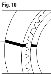
FIGURA 9 Inserire l'apposito attrezzo di bloccaggio della puleggia della pompa di iniezione Q. FIGURA 10 Controllare il corretto allineamento delle tacche di fase R. FIGURA 11 Inserire gli appositi attrezzi di bloccaggio della puleggia della pompa di iniezione S.
