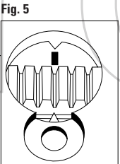
FIGURA 5 Marcas de referencia sobre el volante de inercia del motor. Verificar la correcta alineación de las marcas de fase I. FIGURA 6 Marcas de referencia sobre el volante de inercia del motor. Verificar la correcta alineación de las marcas de fase L.
