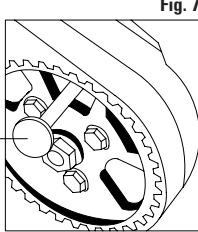
FIGURA 7 Insertar la herramienta específica para inmovilizar la bomba de inyección M.
