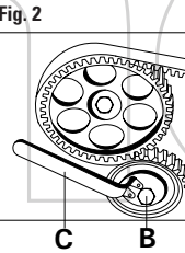
FIGURA 2 Aflojar el tornillo de fijación B, girar el tensor de correa sobre el excéntrico en sentido de las agujas del reloj, utilizando la llave de regulación C. FIGURA 3 Alinear el indicador D del tensor de la correa con la muesca E. Finalmente, apretar el tornillo de fijación B. FIGURA 4 Aflojar el tornillo de fijación F del tensor de correa. Girar el tensor de correa en sentido de las agujas del reloj hasta alinear la marca G con la zona de control H.
