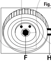
FIGURA 2 Aflojar el tornillo de fijación B, girar el tensor de correa sobre el excéntrico en sentido de las agujas del reloj, utilizando la llave de regulación C. FIGURA 3 Alinear el indicador D del tensor de la correa con la muesca E. Finalmente, apretar el tornillo de fijación B. FIGURA 4 Aflojar el tornillo de fijación F del tensor de correa. Girar el tensor de correa en sentido de las agujas del reloj hasta alinear la marca G con la zona de control H.
