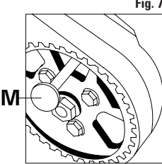
FIGURA 7 Inserire l'apposito attrezzo di bloccaggio della pompa di iniezione M.
