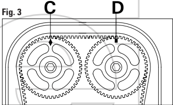
FIGURA 1 Verificar la correcta alineación de los árboles de leva A. FIGURA 2 Verificar el posicionamiento correcto la herramienta de inmovilización de árbol de levas B. FIGURA 3 Verificar el posicionamiento correcto de las marcas de fase C y D.
