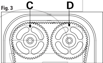
FIGURA 1 Controllare il corretto allineamento degli alberi a camme A. FIGURA 2 Controllare il corretto posizionamento dell'attrezzo di bloccaggio dagli alberi a camme B. FIGURA 3 Controllare il corretto posizionamento delle tacche di fase C e D.
