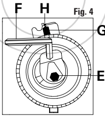
FIGURA 4 Aflojar el tornillo de fijación E del tensor de correa. Actuando con la llave hexagonal F sobre el excéntrico de regulación, girar el tensor de la correa en sentido de las agujas del reloj hasta que el indicador G y la marca H estén alineados. Por último, apriete el tornillo de fijación del tensor.
