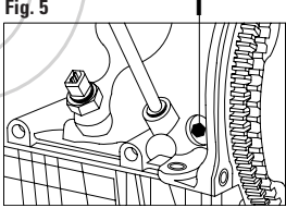
FIGURA 5 Togliere il tappo cieco I dal blocco cilindri. FIGURA 6 Inserire l'apposito attrezzo di bloccaggio dell'albero motore L.
