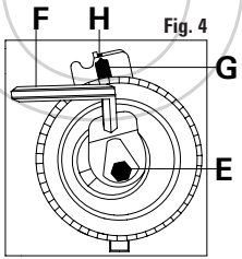
FIGURA 4 Allentare il bullone di bloccaggio E del tendicinghia; ruotare quest'ultimo in senso orario, utilizzando la chiave esagonale F sull'eccentrico di registro. Allineare l'indicatore G del tendicinghia con la tacca H e serrare, quindi, il bullone di bloccaggio E.
