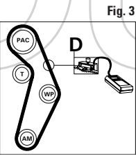
FIGURA 2 Allentare il bullone di bloccaggio B e ruotare in senso antiorario il tendicinghia sull'eccentrico di registro C fino alla corretta tensione; serrare quindi il bullone di bloccaggio B. FIGURA 3 Inserire l'apposito attrezzo di misura del tensionamento D, nel punto indicato, ed agire sul tendicinghia fino al valore di 30 unità SEEM.
