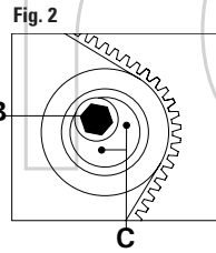
FIGURA 2 Aflojar el tornillo de fijación B, girar el tensor de correa sobre el excéntrico de regulación C en sentido contrario a las agujas de reloj hasta lograr la tensión correcta. Luego vuelva apretar el tornillo de fijación B.
