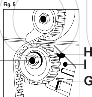
FIGURA 5 Allentare il bullone di bloccaggio F, agendo nel punto indicato, G, del tenditore automatico; portare l'indicatore mobile, H, nella posizione di massima tensione, e, dopo aver fatto coincidere il punto H con il Punto I, serrare il bullone di bloccaggio F.
