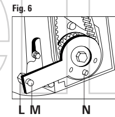
FIGURA 6 Smontare il bullone della pompa dell'olio L e installare al suo posto il prigioniero dell'attrezzo di bloccaggio M. Ruotare l'albero motore fino al PMS del cilindro N° 1 e verificare il corretto posizionamento del grano della puleggia dell'albero motore N. FIGURA 7 Inserire l'apposito attrezzo di bloccaggio dell'albero motore O. FIGURA 8 Inserire l'apposito attrezzo di bloccaggio del volano P.
