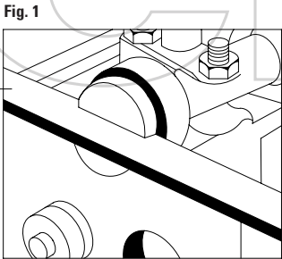
FIGURA 1 Inserire l'apposito attrezzo di bloccaggio dell'albero a camme A. FIGURA 2 Inserire l'apposito attrezzo di bloccaggio dell'albero a camme B.
