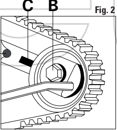
FIGURA 2 Allentare il bullone di bloccaggio B e ruotare il tendicinghia in senso antiorario; allineare l'indicatore C al centro della zona di controllo D e serrare, quindi, il bullone di bloccaggio B.
