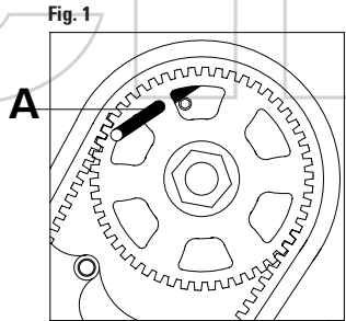
FIGURA 1 Inserire l'apposito attrezzo di bloccaggio dell'albero a camme A.
