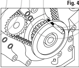
FIGURA 4 Ruotare l'albero motore fino ad allineare il foro per la messa in fase del motore ed installare, quindi, l'apposito attrezzo di bloccaggio F.
