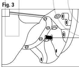
FIGURA 3 Insertar la herramienta de inmovilización del volante motor E. FIGURA 4 Girar el cigüeñal hasta alinear el orificio para la puesta en fase del motor y proceder a instalar la herramienta especial de inmovilización F.
