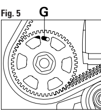
FIGURA 5 Insertar la herramienta específica para inmovilizar la polea de la bomba de inyección G.
