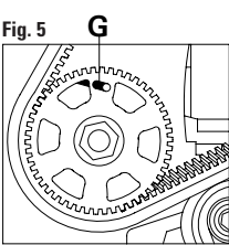
FIGURA 5 Inserire l'apposito attrezzo di bloccaggio della pompa di iniezione G.
