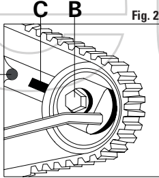
FIGURA 2 Aflojar el tornillo de fijación B, girar el tensor de correa en sentido contrario a las agujas del reloj, alinear el indicador C en el centro de la zona de control D. Luego proceda apretar el tornillo de fijación B.
