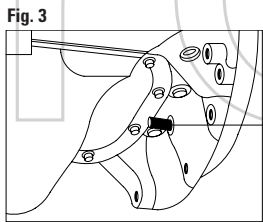
FIGURA 3 Inserire l'apposito attrezzo di bloccaggio del volano E.
