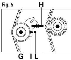
FIGURA 5 Allentare il bullone di bloccaggio G ed inserire l'apposito attrezzo di tensionamento H; portare l'indicatore mobile I, nella posizione di massima tensione, e, dopo aver fatto coincidere il punto I con il Punto L, serrare il bullone di bloccaggio G.
