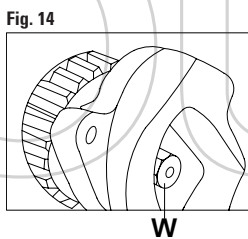
FIGURA 14 Allentare il bullone di bloccaggio W posto sul retro del tendicinghia del contralbero.
