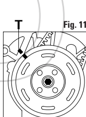
FIGURA 11 Controllare il corretto allineamento delle tacche di fase T.
