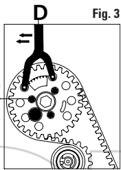
FIGURA 1 Inserire l'apposito attrezzo di bloccaggio dell'albero a camme A. FIGURA 2 Controllare il corretto allineamento della tacca di fasatura verificando che essa sia allineata con l'intaglio sul mozzo del pignone dell'albero a camme: B per motori 4 cilindri e C per motori 3 cilindri. FIGURA 3 Inserire l'apposito attrezzo D, per mantenere gli ingranaggi in tensione e serrare le 3 viti E, sfalsate di 120° l'una dall'altra.
