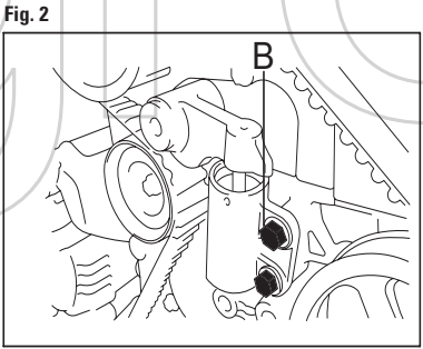
FIGURA 2 Aflojar los tornillos de fijación B del tensor de la correa, demontar las courroies de la distribución.
