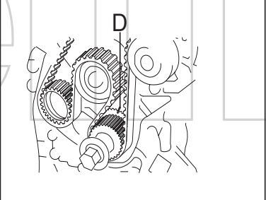
FIGURA 4 Controllare il corretto allineamento della tacca di fase D.
