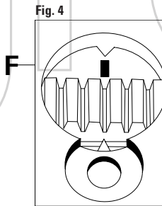
FIGURA 4 Segni di riferimento sul volano: verificare il corretto allineamento delle tacche di fase F.
