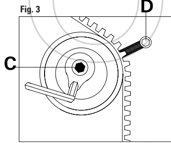
FIGURA 3 Aflojar el tornillo de fijación C. Suelte el tensor de correa hasta la obtener la tensión correcta. Apretar el tornillo de fijación C. Asegurarse que el resorte D quede insertado con su respectivo tornillo de fijación.
