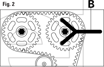
FIGURA 1 Inserire l'apposito attrezzo di bloccaggio dell'albero a camme A. FIGURA 2 Inserire l'apposito attrezzo di bloccaggio B, per mantenere gli ingranaggi in tensione.
