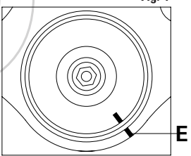
FIGURA 4 Verificar la correcta alineación de las marcas de puesta en fase E.
