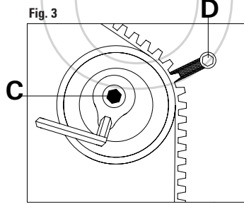
FIGURA 3 Allentare il bullone di bloccaggio C e rilasciare il tendicinghia fino alla corretta tensione, quindi serrare il bullone di bloccaggio C. Assicurarsi che sia inserita la molla D con l'apposito perno di fissaggio.
