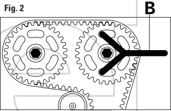
FIGURA 1 Insertar la herramienta especial de inmovilización de árbol de levas A. FIGURA 2 Insertar la herramienta especial de inmovilización B para mantener la correa y los engranajes en tensión.
