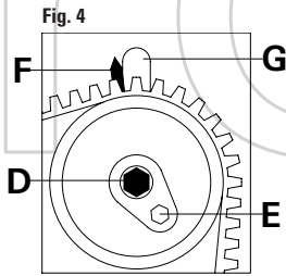
FIGURA 4 Allentare il bullone di bloccaggio D e ruotare in senso orario il tendicinghia sull'eccentrico di registro E; allineare l'indicatore F con la tacca di fase G, serrare quindi il bullone di bloccaggio D. FIGURA 5 Allentare il bullone di bloccaggio I e ruotare in senso orario il tendicinghia sull'eccentrico di registro H; allineare l'indicatore L con la tacca di fase M e serrare, quindi, il bullone di bloccaggio I.
