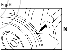
FIGURA 6 Controllare il corretto allineamento delle tacche di fase N. FIGURA 7 Controllare il corretto allineamento delle tacche di fase O.
