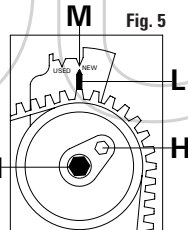
FIGURA 4 Allentare il bullone di bloccaggio D e ruotare in senso orario il tendicinghia sull'eccentrico di registro E; allineare l'indicatore F con la tacca di fase G, serrare quindi il bullone di bloccaggio D. FIGURA 5 Allentare il bullone di bloccaggio I e ruotare in senso orario il tendicinghia sull'eccentrico di registro H; allineare l'indicatore L con la tacca di fase M e serrare, quindi, il bullone di bloccaggio I.
