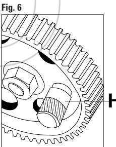
FIGURA 6 Insertar la herramienta para inmovilización de polea de bomba de inyección H. FIGURA 7 Insertar la herramienta para inmovilización de polea de bomba de inyección I.
