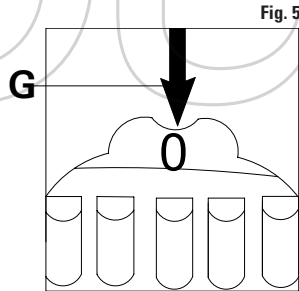
FIGURA 4 Segni di riferimento sul volano: verificare il corretto allineamento delle tacche di fase F. FIGURA 5 Segni di riferimento sul volano: verificare il corretto allineamento delle tacche di fase G.
