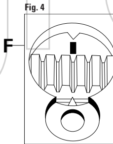
FIGURA 4 Marcas de referencia sobre el volante de inercia del motor: Verificar la correcta alineación de las marcas de fase F. FIGURA 5 Marcas de referencia sobre el volante de inercia del motor: Verificar la correcta alineación de las marcas de fase G.
