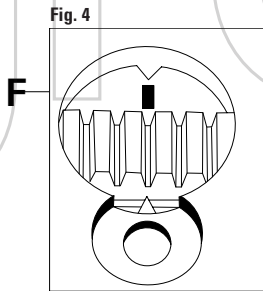
FIGURA 4 Marcas de referencia sobre el volante de inercia del motor: Verificar la correcta alineación de las marcas de fase F. FIGURA 5 Marcas de referencia sobre el volante de inercia del motor: Verificar la correcta alineación de las marcas de fase G.
