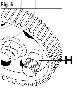
FIGURA 6 Insertar la herramienta para inmovilización de polea de bomba de inyección H. FIGURA 7 Insertar la herramienta para inmovilización de polea de bomba de inyección I.
