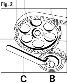
FIGURA 3 Alinear el indicador D del tensor de la correa con la muesca E. Finalmente, apretar el tornillo de fijación B. FIGURA 2 Aflojar el tornillo de fijación B, girar el tensor de correa sobre el excéntrico en sentido de las agujas del reloj, utilizando la llave de regulación C.
