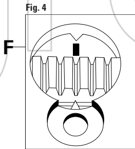
FIGURA 4 Segni di riferimento sul volano: verificare il corretto allineamento delle tacche di fase F. FIGURA 5 Segni di riferimento sul volano: verificare il corretto allineamento delle tacche di fase G.
