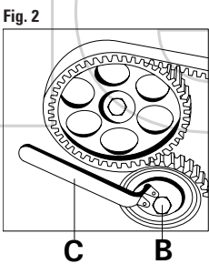
FIGURA 2 Allentare il bullone di bloccaggio B e ruotare in senso orario il tendicinghia utilizzando la chiave C agendo sull'eccentrico di registro.
