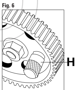
FIGURA 6 Inserire l'apposito attrezzo di bloccaggio della puleggia della pompa di iniezione H. FIGURA 7 Inserire l'apposito attrezzo di bloccaggio della puleggia della pompa di iniezione I.
