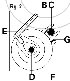
FIGURA 2 Asegurarse que la lamina B este fijada por debajo del tornillo de fijación C. Luego aflojar el tornillo de fijación D, y girar el tensor de la correa sobre el excéntrico de regulación en sentido de las agujas del reloj utilizando para ello la llave hexagonal E hasta lograr la alineación de la marca F con la muesca G. Por último, apretar el tornillo de fijación D.
