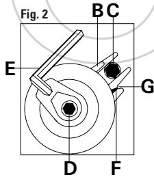
FIGURA 2 Assicurarsi che la piastra B sia fissata al di sotto del bullone di bloccaggio C; allentare il bullone di blocco D e ruotare in senso orario il tendicinghia utilizzando la chiave esagonale E sull'eccentrico di registro; allineare l'indicatore F con la tacca G e serrare; quindi, il bullone di bloccaggio D.
