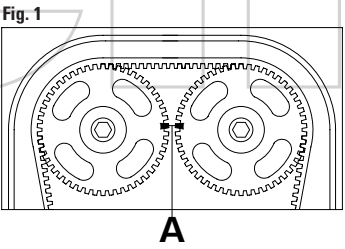
FIGURA 1 Controllare il corretto allineamento delle tacche di fase A.
