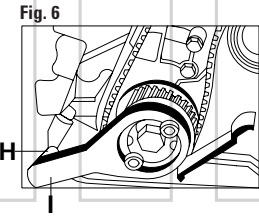
FIGURA 6 Extraer el tornillo del cárter frontal H e insertar la herramienta específica para inmovilizar el cigüeñal I. FIGURA 7 Verificar la correcta alineación de las marcas de puesta en fase L.
