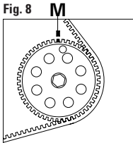
FIGURA 8 Verificar la correcta alineación de las marcas de fase M.
