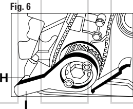
FIGURA 6 Smontare il bullone del carter frontale H ed inserire l'apposito attrezzo di bloccaggio dell'albero motore I. FIGURA 7 Controllare il corretto allineamento delle tacche di fase L.
