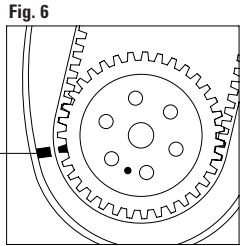
FIGURA 6 Verificar la correcta alineación de las marcas de fase M.
