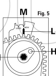
FIGURA 4 Allentare il bullone di bloccaggio D e ruotare in senso orario il tendicinghia sull'eccentrico di registro E; allineare l'indicatore F con la tacca di fase G, serrare quindi il bullone di bloccaggio D. FIGURA 5 Allentare il bullone di bloccaggio I e ruotare in senso orario il tendicinghia sull'eccentrico di registro H; allineare l'indicatore L con la tacca di fase M e serrare, quindi, il bullone di bloccaggio I.
