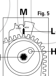
FIGURA 4 Aflojar el tornillo de fijación D. Girar el tensor de la correa sobre el excéntrico de regulación E, en sentido de las agujas del reloj, hasta lograr que el indicador F quede alineado con la muesca de fase G. Por último, apretar el tornillo de fijación D. FIGURA 5 Aflojar el tornillo de fijación I. Girar el tensor de la correa sobre el excéntrico de regulación H en sentido de las agujas del reloj. Luego, alinear el indicador L con la muesca de fase M. Por último apretar el tornillo de fijación I.
