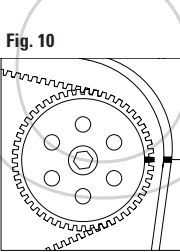
FIGURA 10 Controllare il corretto allineamento delle tacche di fase M (pompa Bosch). FIGURA 11 Controllare il corretto allineamento delle tacche di fase N (pompa Lucas). FIGURA 12 Inserire l'apposito attrezzo di bloccaggio della pompa di iniezione O.
