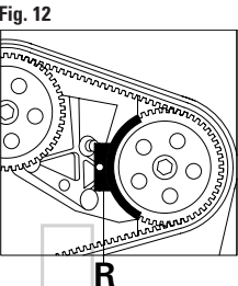
FIGURA 11 Verificar la correcta alineación de las marcas de fase Q. FIGURA 12 Insertar la herramienta para inmovilización de polea de bomba de inyección R.
