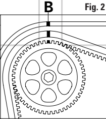
FIGURA 1 Verificar que la marca de puesta a tiempo este en línea con la marca del cárter de la distribución A. FIGURA 2 Verificar la correcta alineación de las marcas de puesta en fase B.
