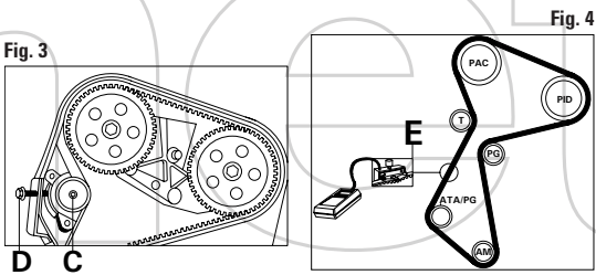
FIGURA 3 Allentare il bullone di bloccaggio C e inserire l'apposito attrezzo di tensionamento D, avvitandolo fino alla corretta tensione; serrare quindi il bullone di bloccaggio C. FIGURA 4 Inserire l'apposito attrezzo di misura del tensionamento E, nel punto indicato, ed agire sul tendicinghia fino ad un valore compreso tra 42.3 e 51.7 unità SEEM (per modello Renault Kangoo); 37 unità SEEM (per modello Renault Espace); 61 ± 5 Hz (per modello Volvo S40). FIGURA 5 Allentare il bullone di bloccaggio F e ruotare in senso antiorario il tendicinghia utilizzando la chiave esagonale G, fino ad allineare le tacche di fase H ed I; serrare, quindi, il bullone di bloccaggio F.
