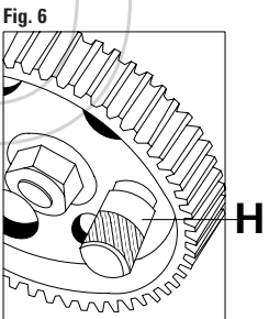
FIGURA 6 Insertar la herramienta para inmovilización de polea de bomba de inyección H. FIGURA 7 Insertar la herramienta para inmovilización de polea de bomba de inyección I.
