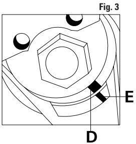
FIGURA 3 Alinear el indicador D del tensor de la correa con la muesca E. Finalmente, apretar el tornillo de fijación B. FIGURA 2 Aflojar el tornillo de fijación B, girar el tensor de correa sobre el excéntrico en sentido de las agujas del reloj, utilizando la llave de regulación C.
