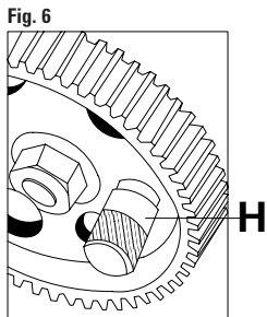
FIGURA 6 Inserire l'apposito attrezzo di bloccaggio della puleggia della pompa di iniezione H. FIGURA 7 Inserire l'apposito attrezzo di bloccaggio della puleggia della pompa di iniezione I.
