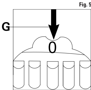
FIGURA 4 Segni di riferimento sul volano: verificare il corretto allineamento delle tacche di fase F. FIGURA 5 Segni di riferimento sul volano: verificare il corretto allineamento delle tacche di fase G.
