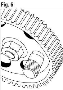
FIGURA 6 Insertar la herramienta para inmovilización de polea de bomba de inyección H. FIGURA 7 Insertar la herramienta para inmovilización de polea de bomba de inyección I. FIGURE 6 Introduire l'outil approprié de blocage poulie pompe d'injection H. FIGURE 7 Introduire l'outil approprié de blocage poulie pompe d'injection I.
