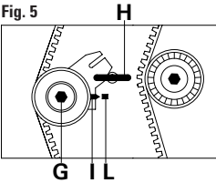
FIGURA 5 Aflojar el tornillo de fijación G. Insertar la herramienta específica H para tensar correas. Llevar el indicador móvil I hasta la posición de máxima tensión, y después de haber hecho coincidir los puntos I y L, apretar el tornillo de fijación G.
