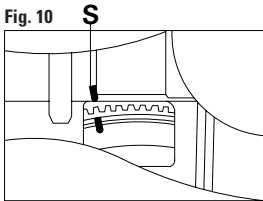
FIGURA 6 Insertar la herramienta específica para inmovilizar el volante motor M. FIGURA 7 Verificar la correcta alineación de las marcas de fase N. FIGURA 8 Desmontar el tornillo de la bomba de aceite O, e instalar en su lugar el prisionero de la herramienta de inmovilización P. Girar el cigüeñal hasta el PMS del cilindro N° 1 y verificar la correcta alineación de la marca de la polea del cigüeñal. FIGURA 9 Insertar la herramienta especial para inmovilización de cigüeñal motor R. FIGURA 10 Marcas de referencia sobre el volante de inercia del motor. Verificar la correcta alineación de las marcas de fase S.
