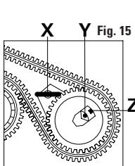
FIGURA 14 Aflojar el tornillo de fijación W situado en la parte posterior del tensor de la correa del árbol balanceador. FIGURA 15 Aflojar el tornillo de fijación W del tensor de correa del árbol balanceador. Insertar la herramienta específica X para tensar correas. Luego, alinear el indicador móvil Y con la muesca de fase Z. Por último, volver a apretar el tornillo de fijación W.
