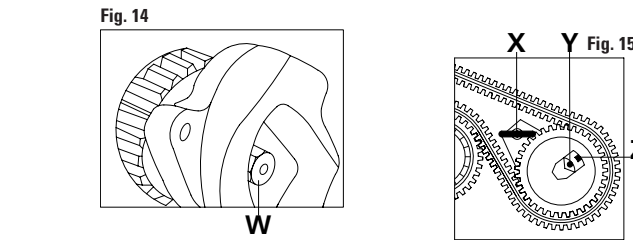
FIGURA 14 Allentare il bullone di bloccaggio W posto sul retro del tendicinghia del contralbero. FIGURA 15 Allentare il bullone di bloccaggio W del tendicinghia del contralbero ed inserire l'apposito attrezzo di tensionamento X; allineare l'indicatore mobile Y con la tacca di fase Z; serrare, quindi, il bullone di bloccaggio W.
