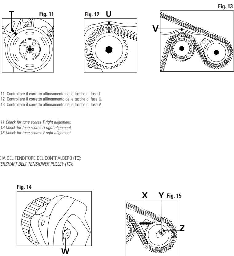
FIGURA 14 Allentare il bullone di bloccaggio W posto sul retro del tendicinghia del contralbero. FIGURA 15 Allentare il bullone di bloccaggio W del tendicinghia del contralbero ed inserire l'apposito attrezzo di tensionamento X; allineare l'indicatore mobile Y con la tacca di fase Z; serrare, quindi, il bullone di bloccaggio W.
