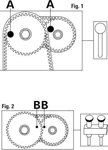
FIGURA 1 Inserire gli appositi attrezzi di bloccaggio degli alberi a camme A. FIGURA 2 Inserire l'apposito attrezzo di bloccaggio degli alberi a camme B.
