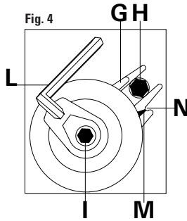
FIGURA 4 Assicurarsi che la piastra G sia fissata al di sotto del bullone di bloccaggio H; allentare il bullone di blocco I e ruotare in senso orario il tendicinghia utilizzando la chiave L sull'eccentrico di registro; allineare l'indicatore M con la tacca N e serrare, quindi, il bullone di bloccaggio I.
