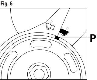
FIGURA 5 Verificar la correcta alineación de la marca de puesta en fase O. FIGURA 6 Verificar la correcta alineación de la marca de puesta en fase P.
