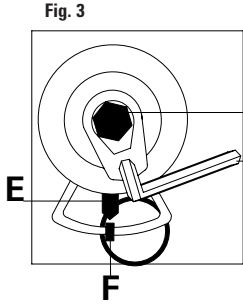
FIGURA 3 Aflojar el tornillo de fijación C. Girar el tensor de correa en sentido contrario a las agujas del reloj, actuando con la llave D sobre el excéntrico de regulación hasta alinear el indicador E con la muesca F. Por último, apretar el tornillo de fijación C.
