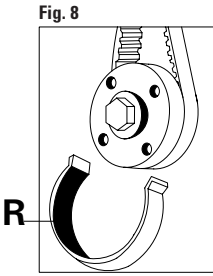
FIGURA 6 Inserire l'apposito attrezzo di bloccaggio del volano P. FIGURA 7 Controllare il corretto allineamento della tacca di fase Q. FIGURA 8 Inserire l'apposito attrezzo di bloccaggio della cinghia di distribuzione R.
