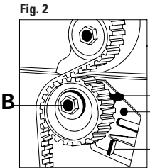
FIGURA 2 Allentare il bullone di bloccaggio B, agendo nel punto indicato C del tenditore, quindi, portare l'indicatore mobile D, nella posizione di massima tensione, e dopo aver fatto coincidere il punto D con il Punto E, serrare il bullone di bloccaggio B.
