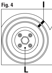
FIGURA 3 Desmontar los tornillos F de la bomba de aceite, y en su lugar, hacer coincidir el punto de centrado G. Luego insertar la herramienta de inmovilización "H".
