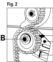
FIGURA 2 Aflojar el tornillo de fijación B. Actuando sobre el punto indicado C del tensor, llevar el indicador móvil D hasta la posición de máxima tensión, y luego de hacer que los puntos D y E coincidan, volver a apretar el tornillo de fijación B.
