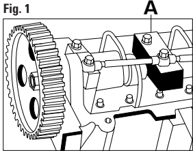
FIGURA 1 Inserire l'apposito attrezzo di bloccaggio dell'albero a camme A, nella posizione N° 2 del cappellotto.
