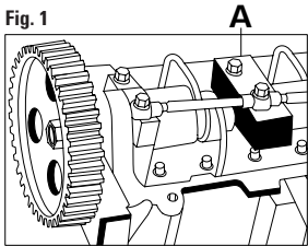
FIGURA 1 Insertar la herramienta especial de inmovilización de árbol de levas A en la posición N° 2 de la copa.
