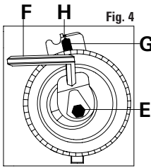
FIGURA 4 Allentare il bullone di bloccaggio E del tendicinghia; ruotare quest'ultimo in senso orario, utilizzando la chiave esagonale F sull'eccentrico di registro. Allineare l'indicatore G del tendicinghia con la tacca H e serrare, quindi, il bullone di bloccaggio E.
