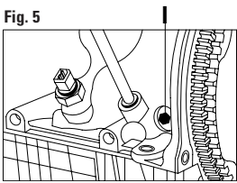
FIGURA 5 Togliere il tappo cieco I dal blocco cilindri. FIGURA 6 Inserire l'apposito attrezzo di bloccaggio dell'albero motore L.
