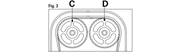
FIGURA 1 Verificar la correcta alineación de los arboles de leva A. FIGURA 2 Verificar el posicionamiento correcto la herramienta de inmovilización de árbol de levas B. FIGURA 3 Verificar el posicionamiento correcto de las marcas de fase C y D.
