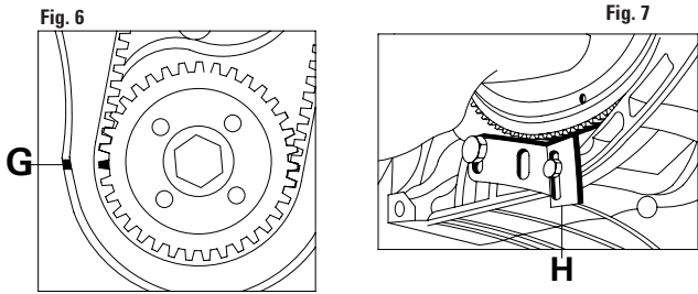
FIGURA 6 Controllare il corretto allineamento delle tacche di fase G. FIGURA 7 Inserire l'apposito attrezzo di bloccaggio del volante H.
