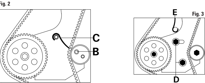
FIGURA 2 Aflojar el tornillo de fijación B, insertar el resorte C del tensor de correa. Quitar las herramientas de bloqueo y girar el cigüeñal 60° en sentido contrario al de las agujas de reloj. Luego vuelva apretar el tornillo de fijación B. FIGURA 3 Aflojar los tornillos de fijación D, insertar el resorte E del tensor de correa, extraer las herramientas de inmovilización y girar el cigüeñal en sentido contrario al de las agujas del reloj aproximadamente 60°. Por ultimo, apretar los tornillos de fijación D.
