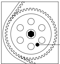
FIGURA 6 Inserire l'apposito attrezzo di bloccaggio della puleggia della pompa di iniezione H.
