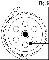
FIGURA 6 Insertar la herramienta para inmovilización de polea de bomba de inyeccion H.
