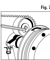
FIGURA 6 Insertar la herramienta para inmovilización del tensor de correa G. FIGURA 7 Girar el tensor de correa en sentido contrario a las agujas del reloj, utilizando para ello la llave hexagonal H, hasta alcanzar la tensión correcta. Por último, desmonte la herramienta de inmovilización G.
