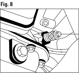
FIGURA 8 Insertar la herramienta especial para inmovilización de cigüeñal motor I.
