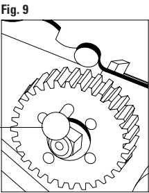
FIGURA 9 Insertar la herramienta para inmovilización de polea de bomba de inyección L.
