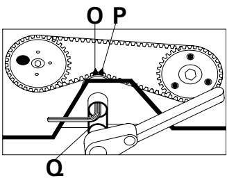
FIGURA 10 Extraer el amortiguador de vibraciones de la polea de la bomba de inyección por medio de los tornillos M. Jamás afloje el tornillo N. FIGURA 11 Aflojar el tornillo de fijación del tensor de correa. Girar el tensor de la correa en sentido contrario a las agujas del reloj hasta que los indicadores O y P estén alineados. Por último, apriete el tornillo de fijación del tensor utilizando la herramienta específica Q.
