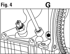
FIGURA 4 Smontare il bullone G ed inserire al suo posto l'attrezzo di bloccaggio H. FIGURA 5 Inserire l'apposito attrezzo di bloccaggio dell'albero motore H e ruotare l'albero motore fino a alla battuta contro il perno.
