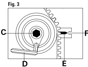
FIGURA 3 Allentare il bullone di bloccaggio C e ruotare in senso orario il tendicinghia, utilizzando la chiave esagonale D, fino ad allineare le tacche di fase E ed F; serrare quindi il bullone di bloccaggio C.
