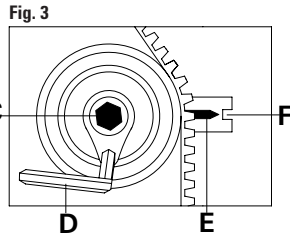
FIGURA 3 Aflojar el tornillo de fijación C. Girar el tensor de correa en sentido de las agujas del reloj, utilizando la llave hexagonal D hasta que las marcas de fase E y F estén en línea. Por último, apretar el tornillo de fijación C.
