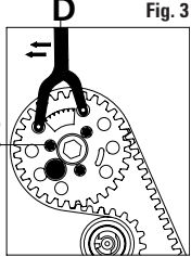
FIGURA 1 Insertar la herramienta especial de inmovilización de árbol de levas A. FIGURA 2 Verificar que la marca de puesta a tiempo este correctamente alineada con la muesca tallada sobre el mozo del piñón del árbol de levas; B para motores 4 cilindros y C para motores 3 cilindros. FIGURA 3 Insertar la herramienta especial D para mantener la correa en tensión entre los engranajes, y apretar los 3 tornillos E, los cuales están distanciados 120° entre sí.
