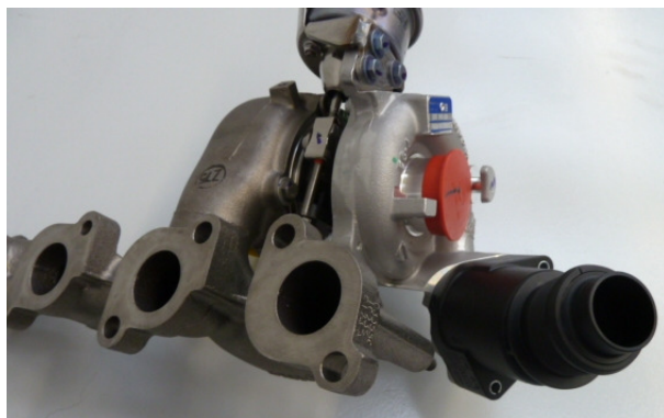
Imaginea 1 Turbosuflantă cu amortizor de zgomot
